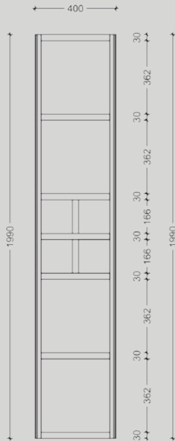
κύρια όψη
