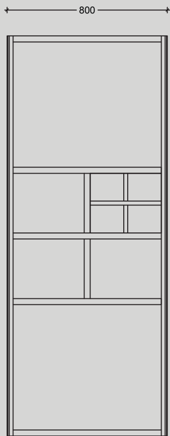
κύρια όψη
