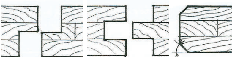
παραδείγματα συναρμολόγησης
